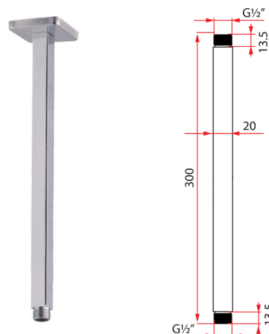
RSA-VAS-300
